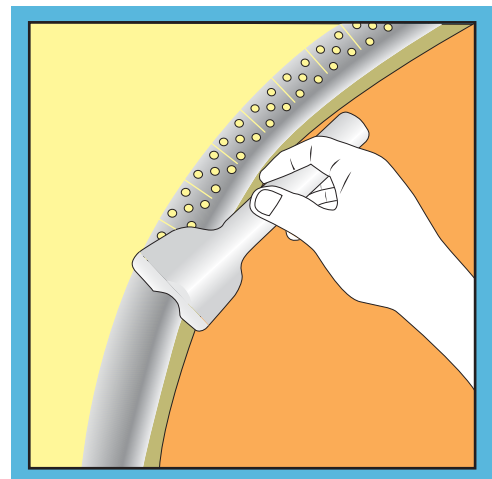
อุปกรณ์เก็บงานคิ้วมุมมนรุ่นตัดโค้ง 19 mm. Bullnose Archway Finishing Tool BAF001
